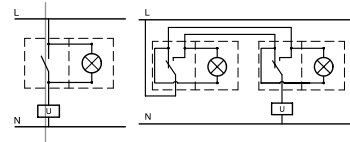
לחיבור אביזר פיקוד לאיתור בחשיכה
