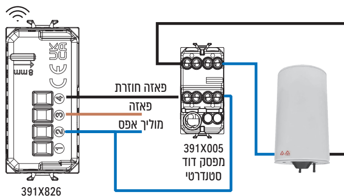
תרשים 1 (חיבור לדוד)
