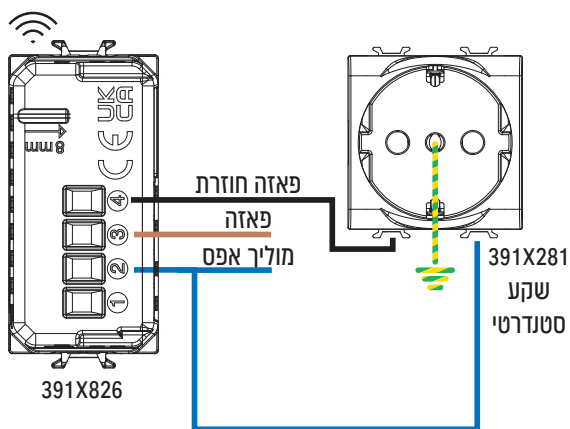
תרשים 2 (חיבור לשקע)
